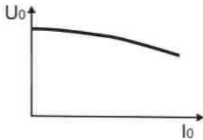
Рис. 8. Внешняя характеристика выпрямителя
