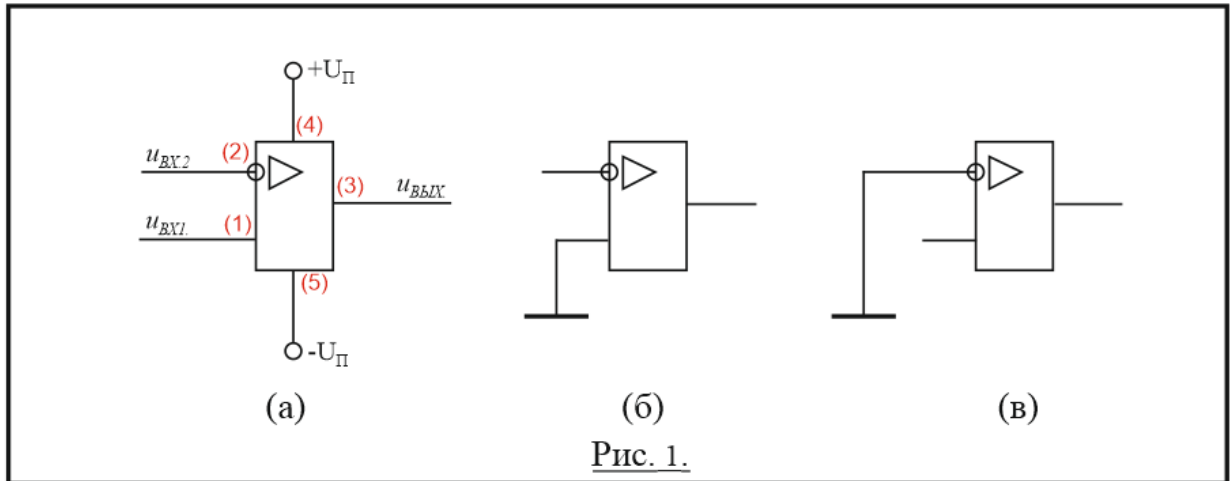
7. Компаратор на ОУ.
